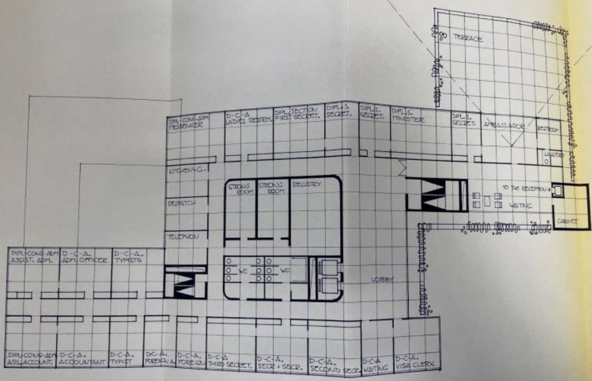
I. OBERGESCHOSS / FIRST FLOOR
